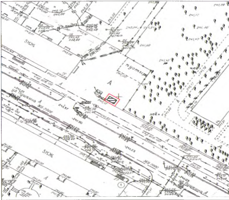
Топографическая основа в масштабе 1:500
