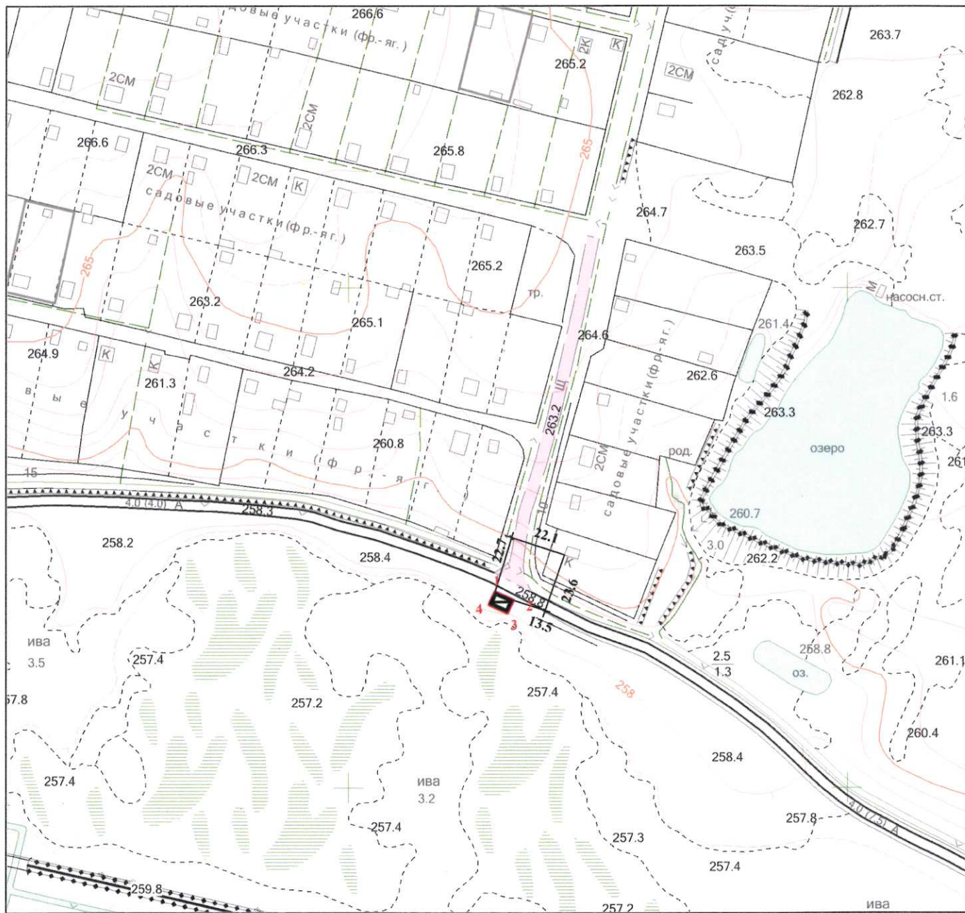
Топографическая основа в масштабе 1:2000
